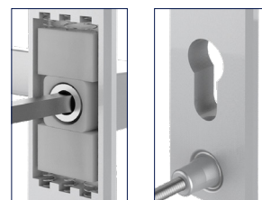
6 MUELLES DE PRESIÓN Y ESCUDO MACIZO
