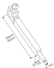
PASADOR ATLAS CON LLAVE
