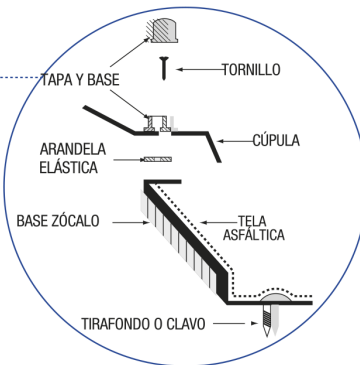
Esquema de Montaje de cúpula sobre base-zócalo.
